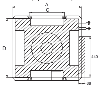
T12H-LC/I, T18H-LC/I
