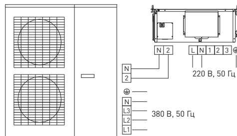
T36H—T60H (3-фазные)
