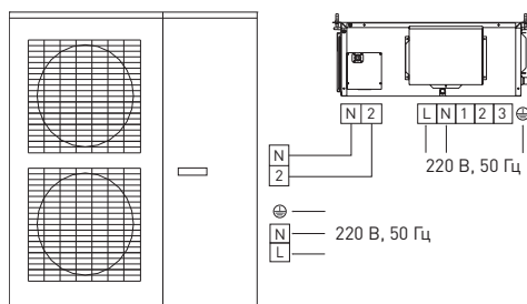
T09H—T36H (1-фазные)
